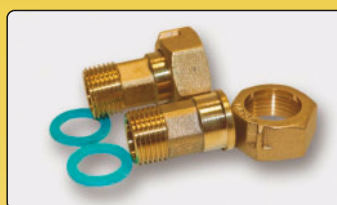
Art. 1522 připojovací šroubení k vodoměrům (sada) 2 matky, 2 niply, vč. těsnění
