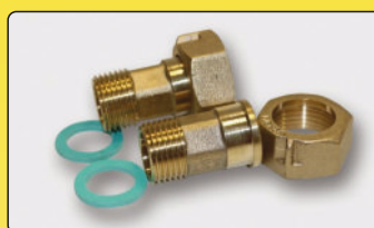
Art. 1522 připojovací šroubení k vodoměrům (sada) 2 matky, 2 niplý, vč. těsnění
